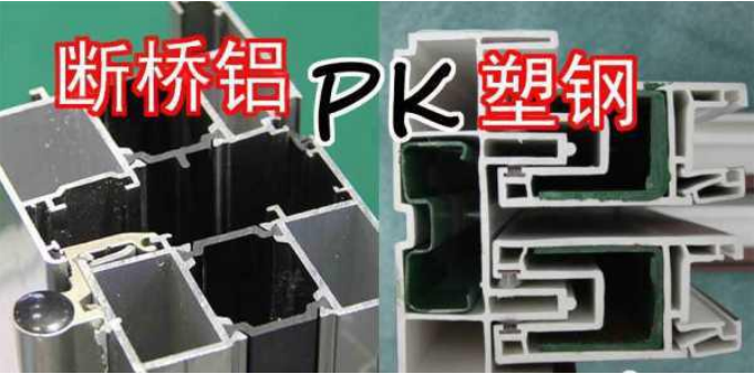
左边断桥铝窗户能清楚看到隔热条，右边塑钢窗能清楚看到绿色的钢衬
