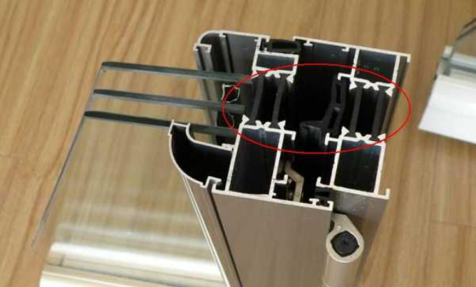
中间黑色的隔热条就是断桥，一般都是尼龙材料
